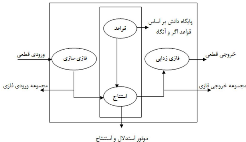
شکل (۱): اجزای پنج‌گانه سیستم‌های فازی
